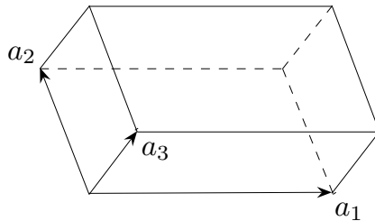
Obr. 1. Objem rovnoběžnostěnu s hranami a_1, a_2, a_3 je roven |\det A| , kde a_1, a_2, a_3 jsou sloupce matice A .
