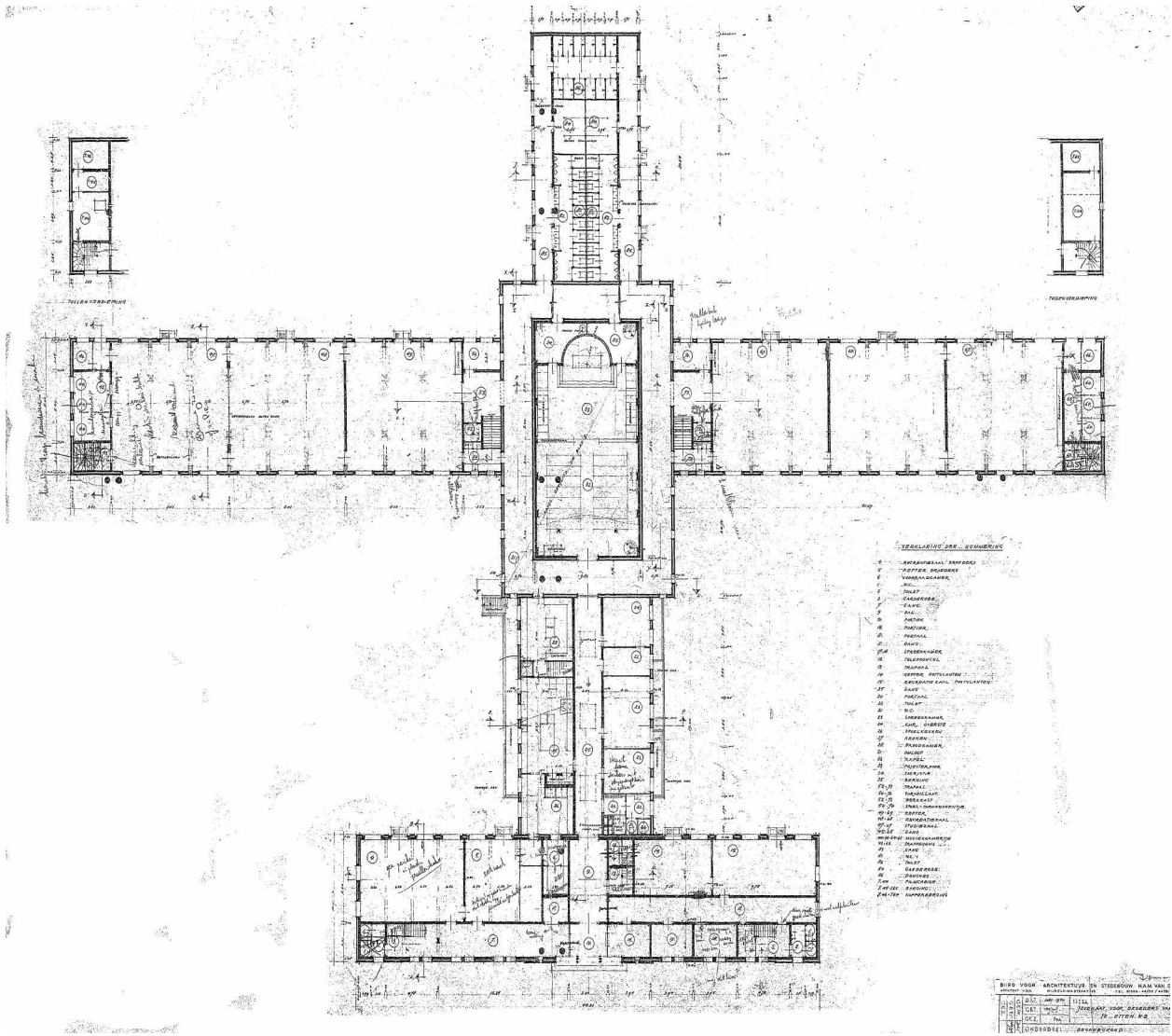
Afb. 1. Plattegrond klooster en juvenaat, mei 1950.
