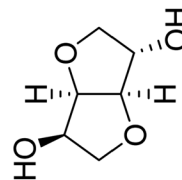
isosorbide
