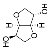
isosorbide
