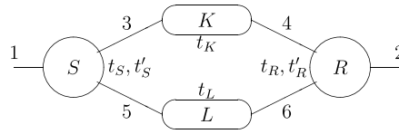
Fig. 1. Connection diagram for PAR protocol.
