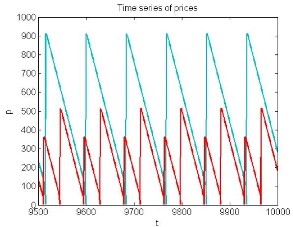
(d) High-period cycle for \lambda = 10
